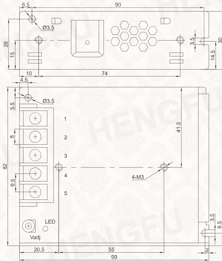
机壳 Frame
